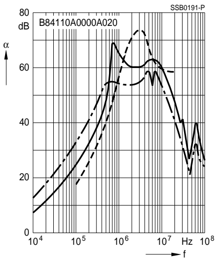
Filter für 2 A
